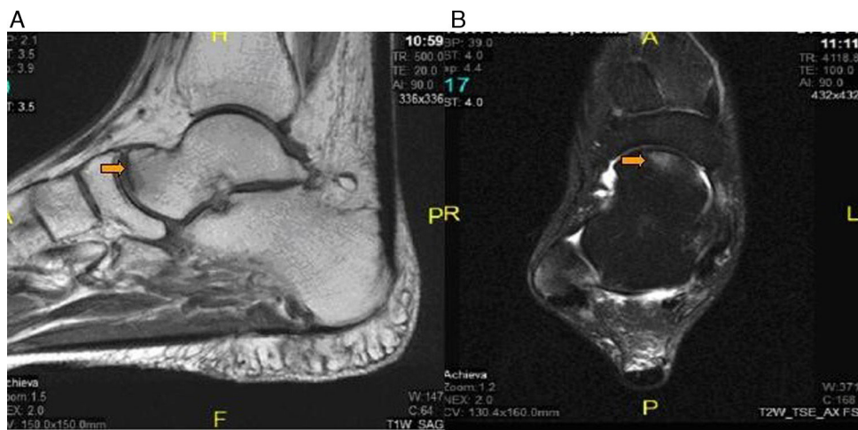
Figura 3. A) RM corte sagital en T1, que muestra lesión focal a nivel de la cabeza astragalina con edema difuso del resto del hueso del pie derecho. B) RM axial del pie en secuencia T2, saturación grasa mostrando: lesión focal a nivel de la cabeza astragalina y derrame articular a nivel de articulación tibio astragalina anterior y posterior del pie derecho.
